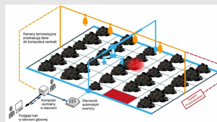
Schemat magazynu, rozmieszczenie kamer i systemów
