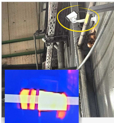
System Monitoringu Rozkładu Temperatur Pieca Obrotowego
