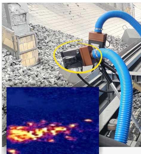
Mobilny Zestaw Termograficzny Monitoringu i Ostrzegania w Koksowni
